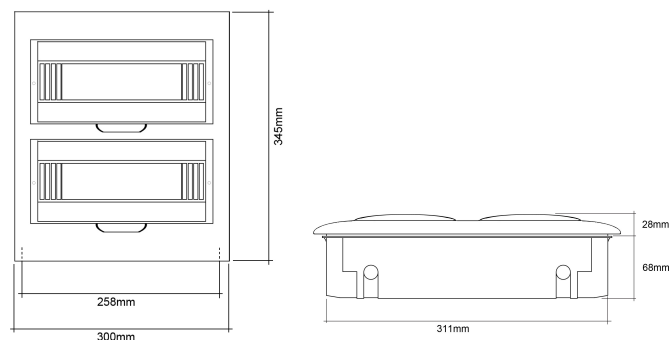
Modelo JNG-24 (24 módulos)
