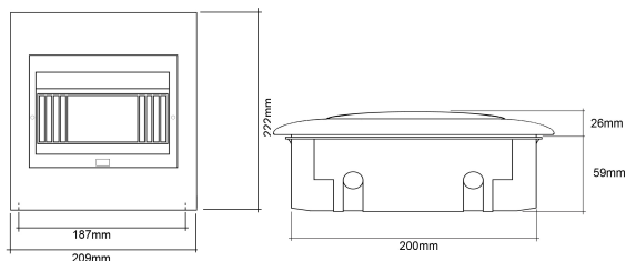
Modelo JNG-08 (8 módulos)
