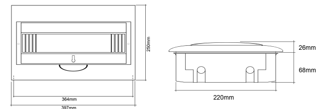
Modelo JNG-18 (18 módulos)
