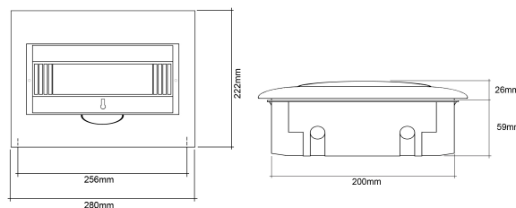
Modelo JNG-12 (12 módulos)
