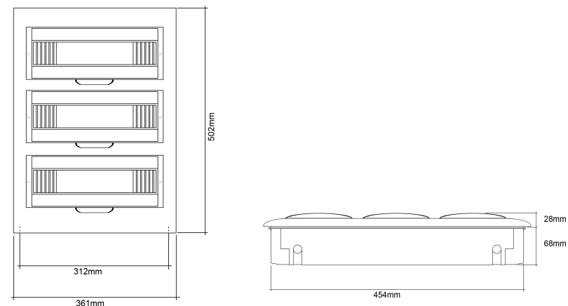
Modelo JNG-36 (36 módulos)
