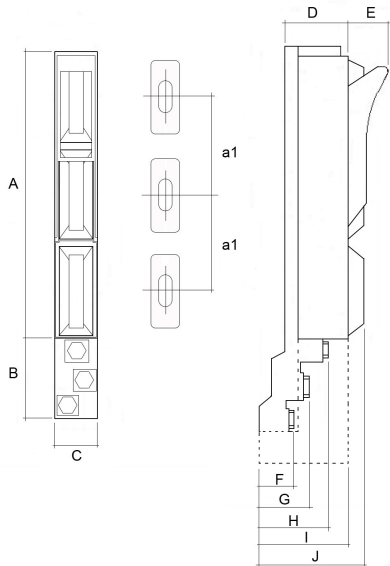
Seccionadora DNH5-160
