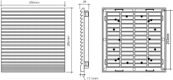
Microventilador 180x180 200x200 220x220 225x225
