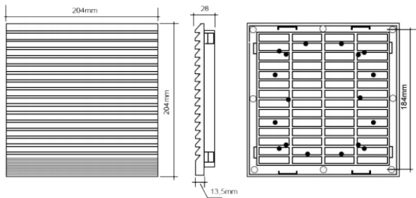
Microventilador 120x120 150x150 170x150
